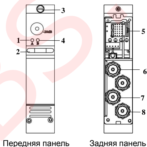
Рис.2 Передняя и задняя панели модуля ВЧ переключателя
