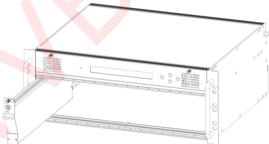
Рис.3 Установка модуля ВЧ переключателя в шасси
